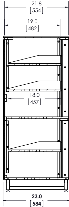
SECTION A-A
